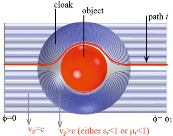
Fig. 12.1 EM wave propagation inside the cloak
